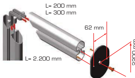
9020070 Soporte lat. tuvo oval Material. Zamac Acabado. Niquel Pz = 1
